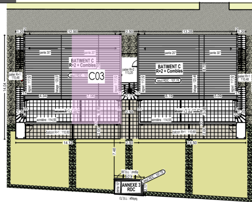
RDC C03 entrée 5.59 séjour-cuisine + PL 27.38 wc 2.60 sde 5.18 chambre 1 9.19 chambre 2 12.01 TOTAL 61.95 terrasse 19.17 jardin 52.19 cellier C03 3.40
